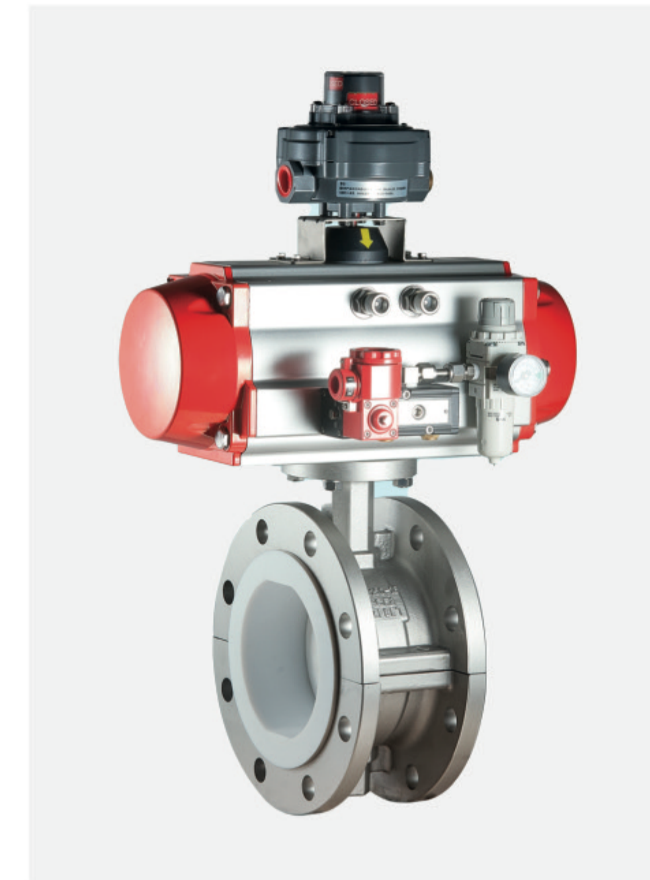
气动衬氟蝶阀
