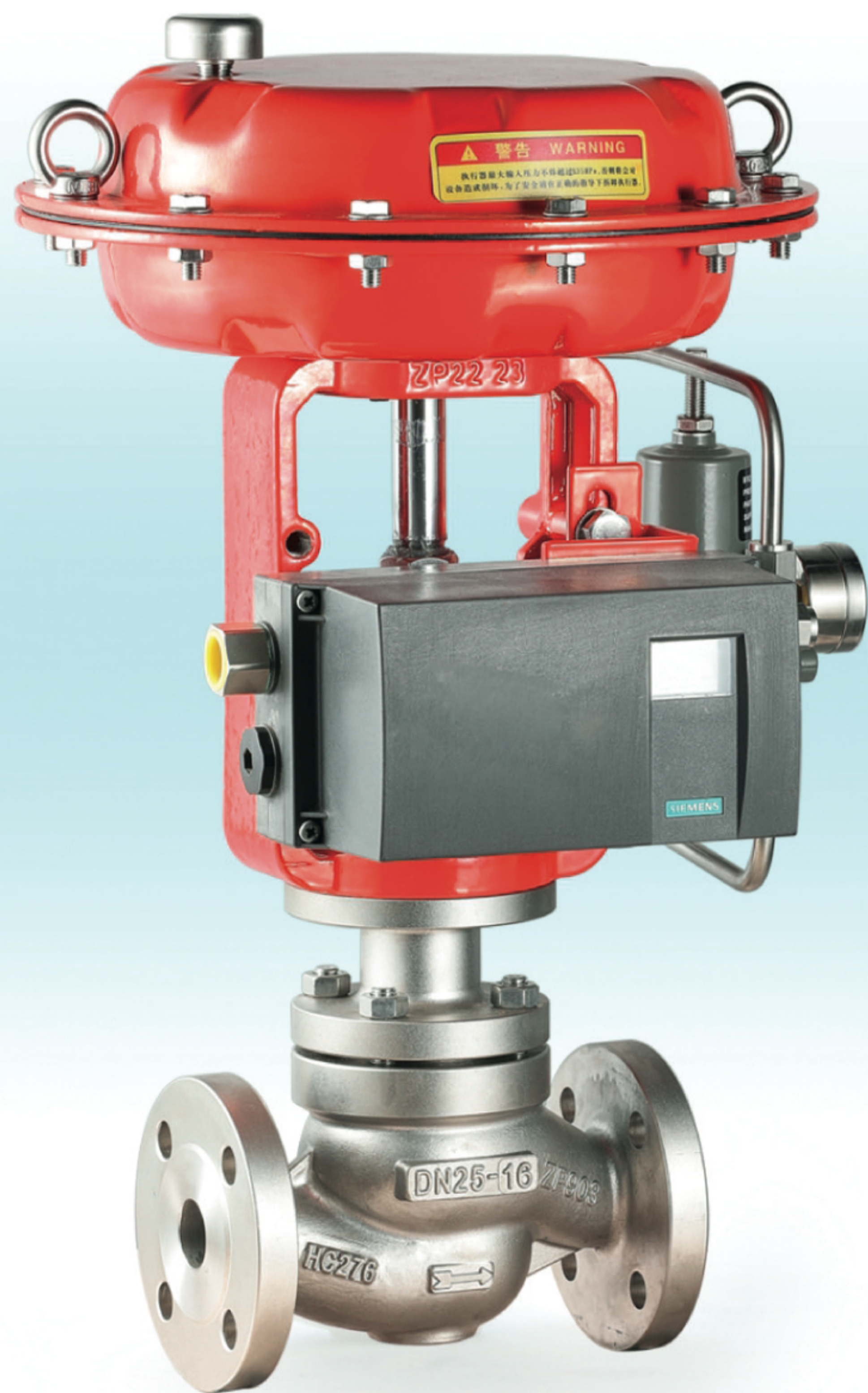
气动调节阀
