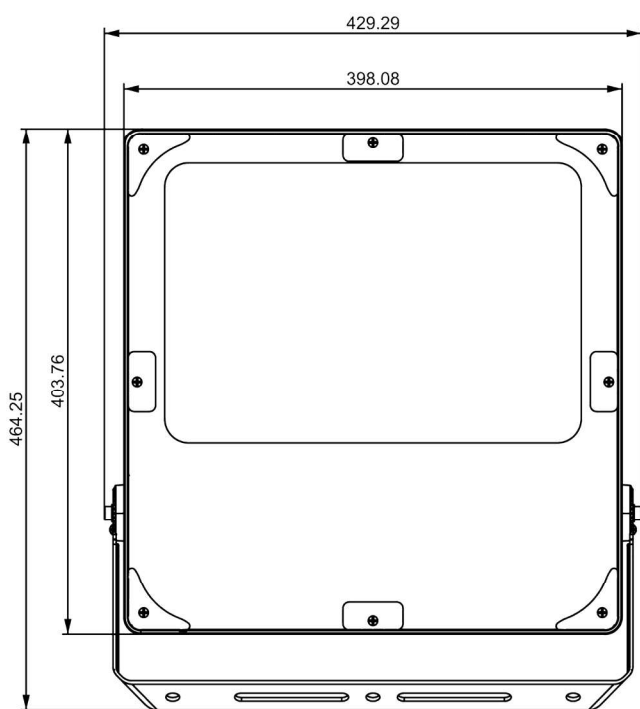
主视图
