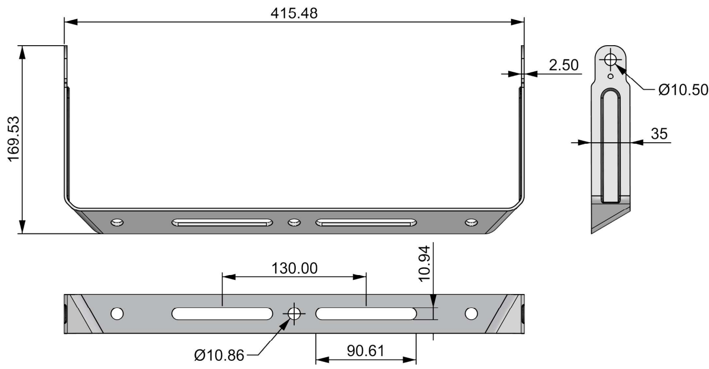
尺寸孔位
