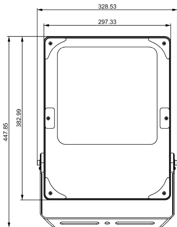
主视图
