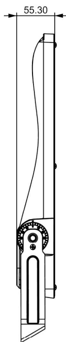
左视图
