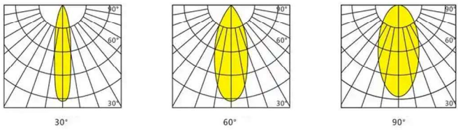
小方块透镜二十四合一 30度60度90度
