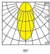
小方块透镜长条形 90度
