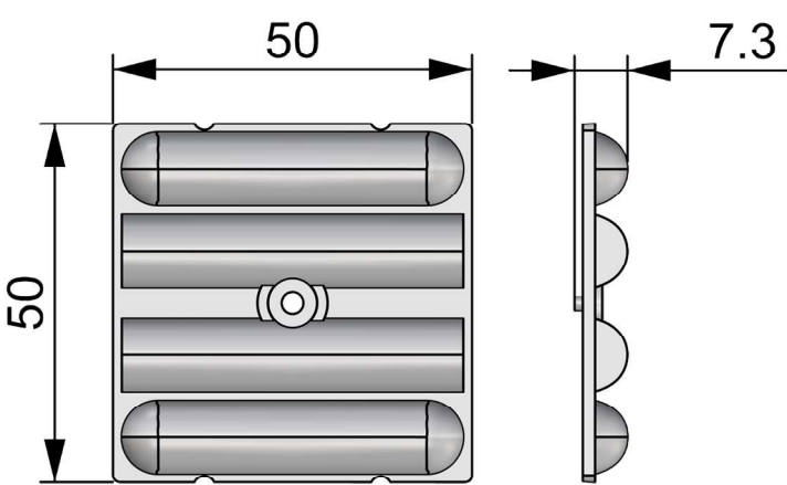
小方块透镜长条形 90度
