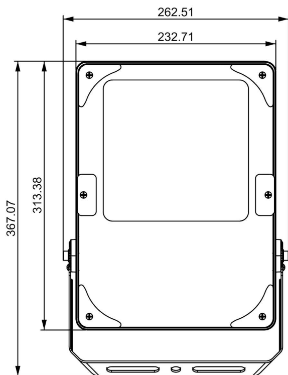
主视图
