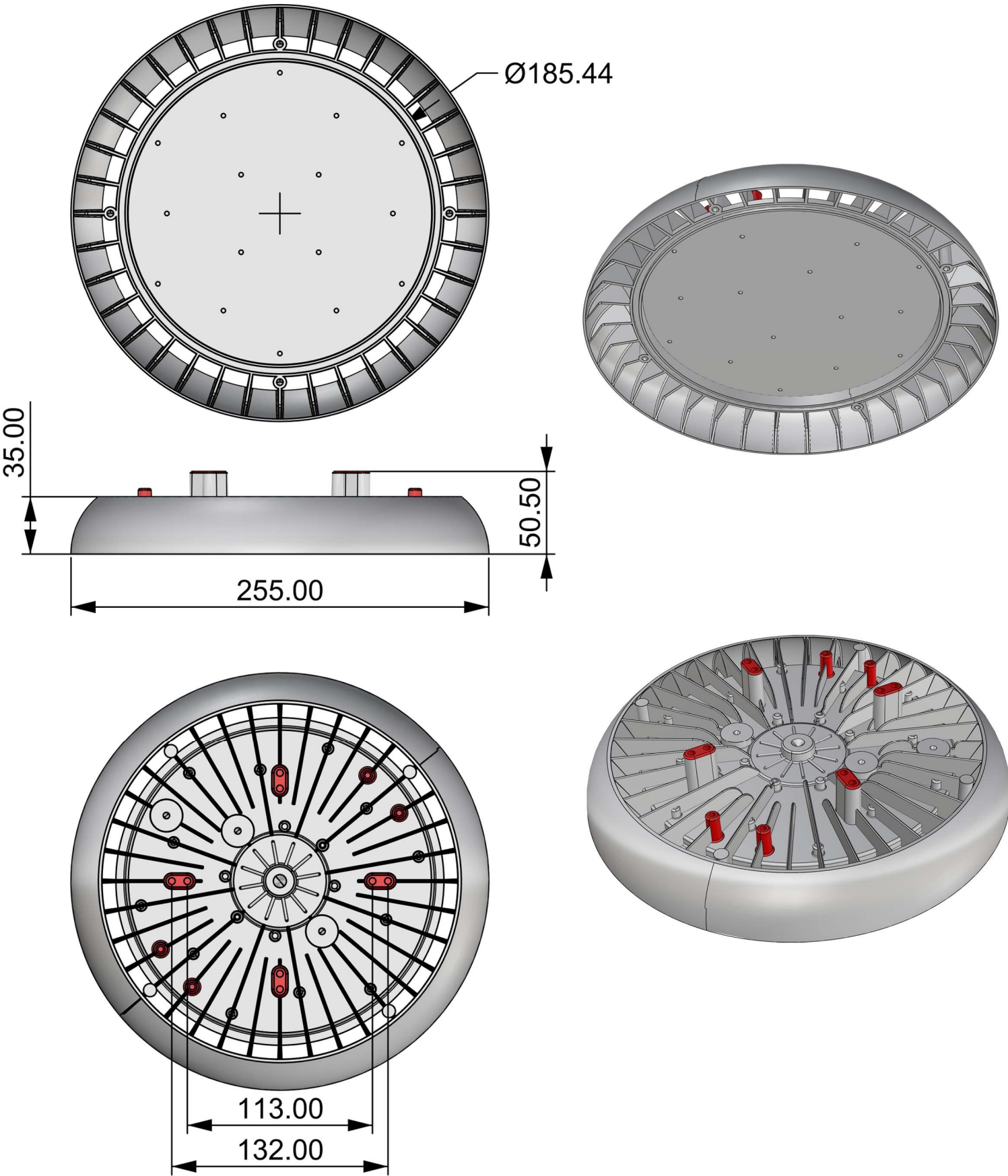
灯体
