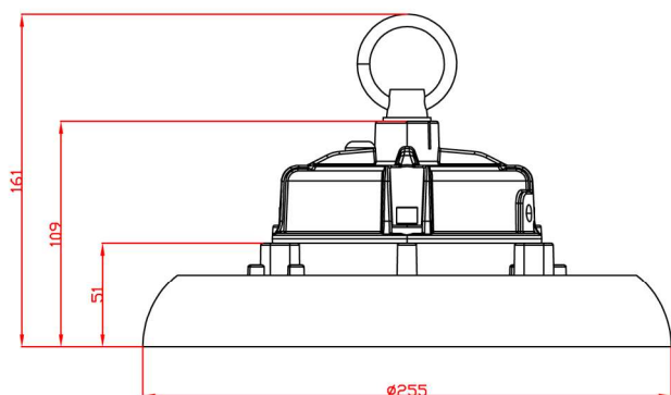
主视图
