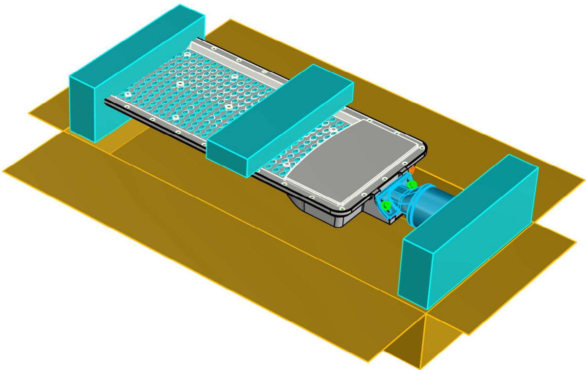
外箱：W280mm*L700mm*H115mm
