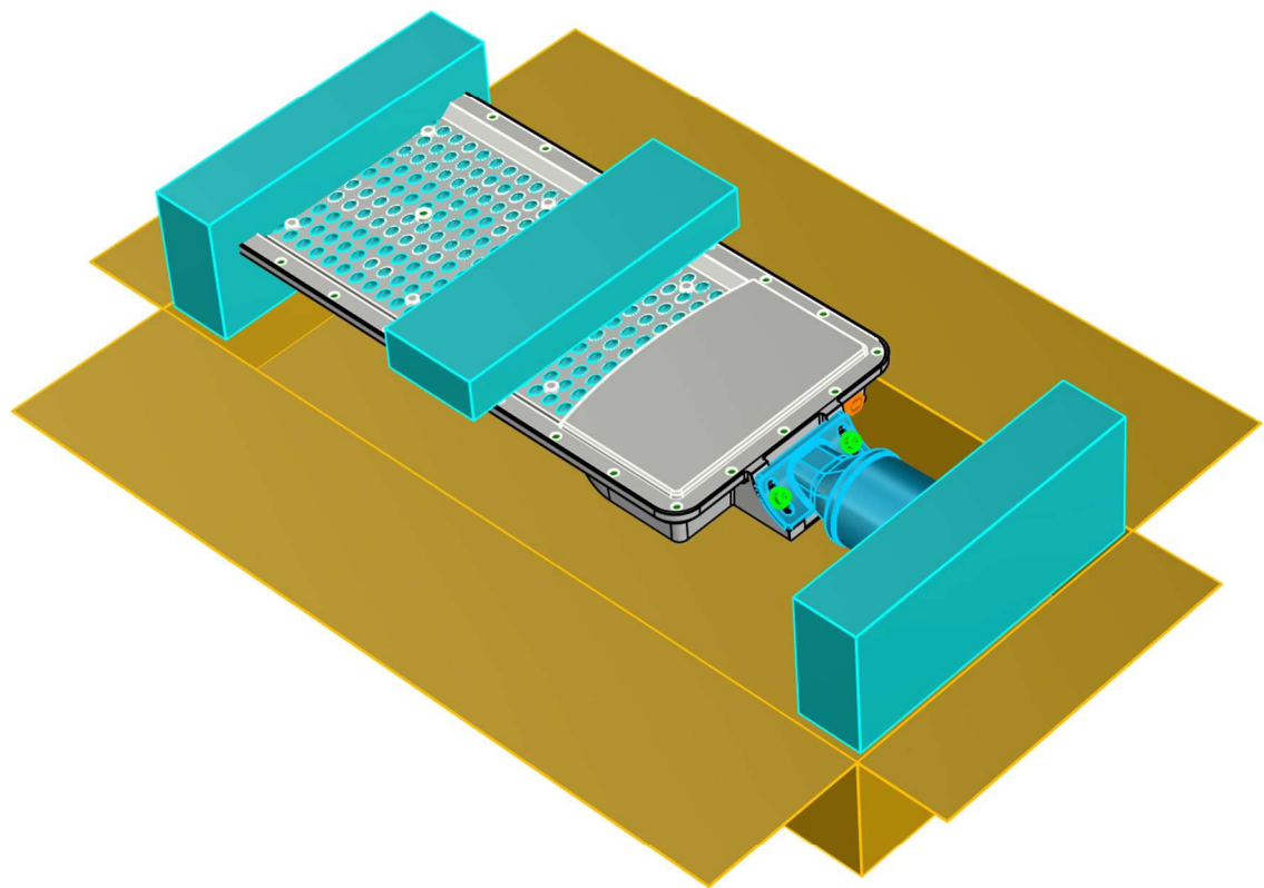
外箱：W265mm*L645mm*H115mm
