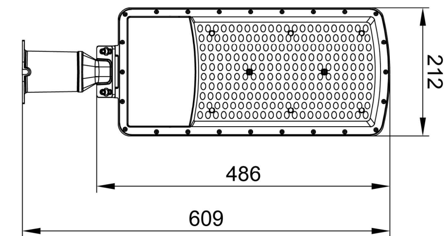
主视图
