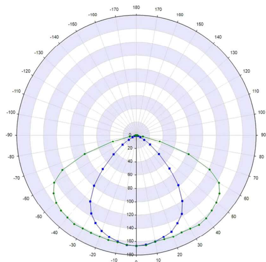
配光曲线
