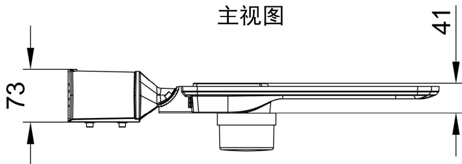
俯视图
