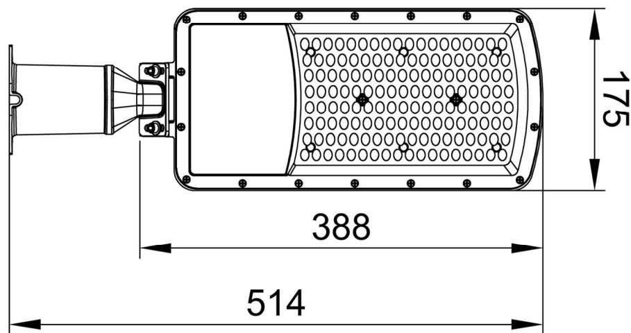
主视图
