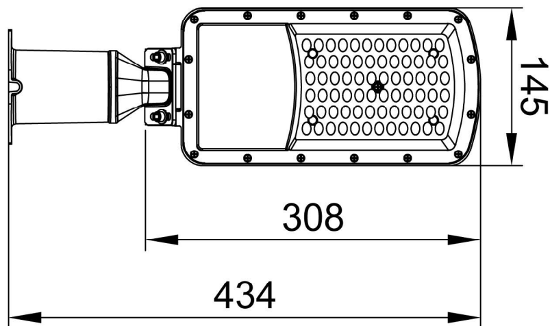
主视图
