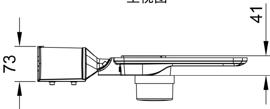
俯视图
