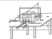
图5 脉冲磁场抗扰度试验接线图
