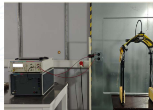
图6 脉冲磁场抗扰度试验受试设备布置图
