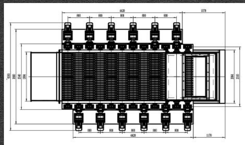
XCDRS滚轴筛香蕉型
