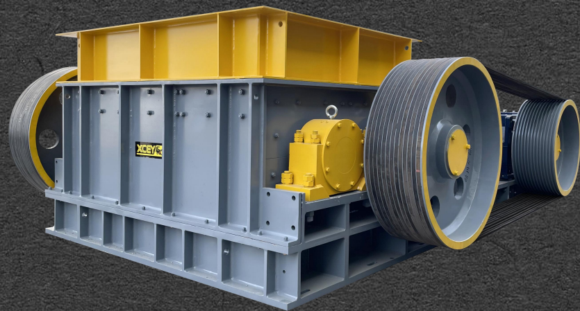
XCMD筛分式破碎机
