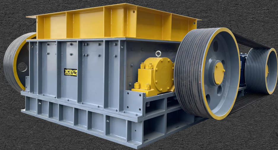
XCMD筛分式破碎机外形图
