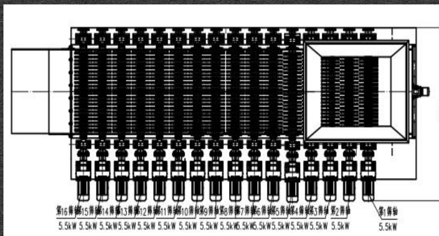
XCDRS滚轴筛阶梯型
