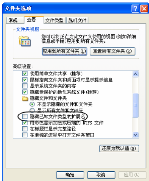
图1-8 扩展名设置
