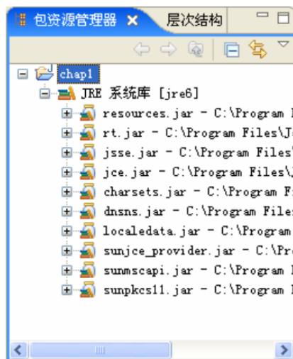
图1-17 项目结构
