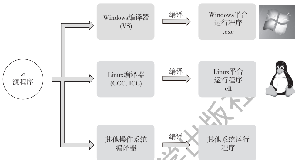
图1-1 C语言编译执行过程
