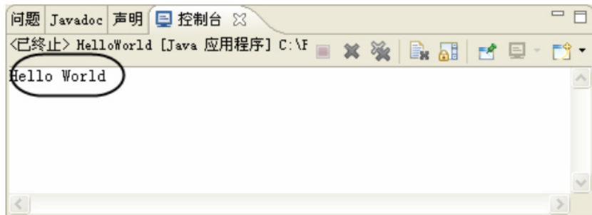
图1-20 运行结果
