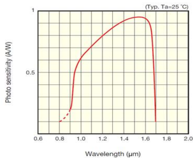
光谱响应曲线
