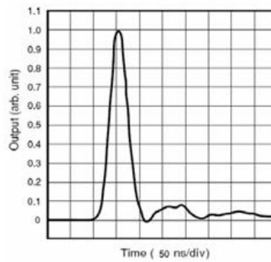
脉冲响应
