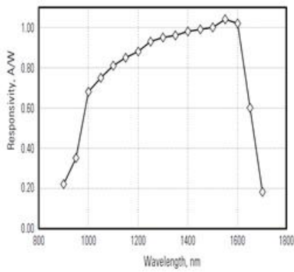
光谱响应
