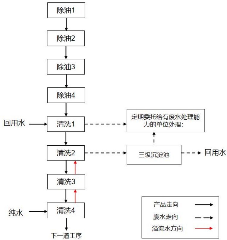
项目产品除油清洗线走向和清洗废水流向示意图
