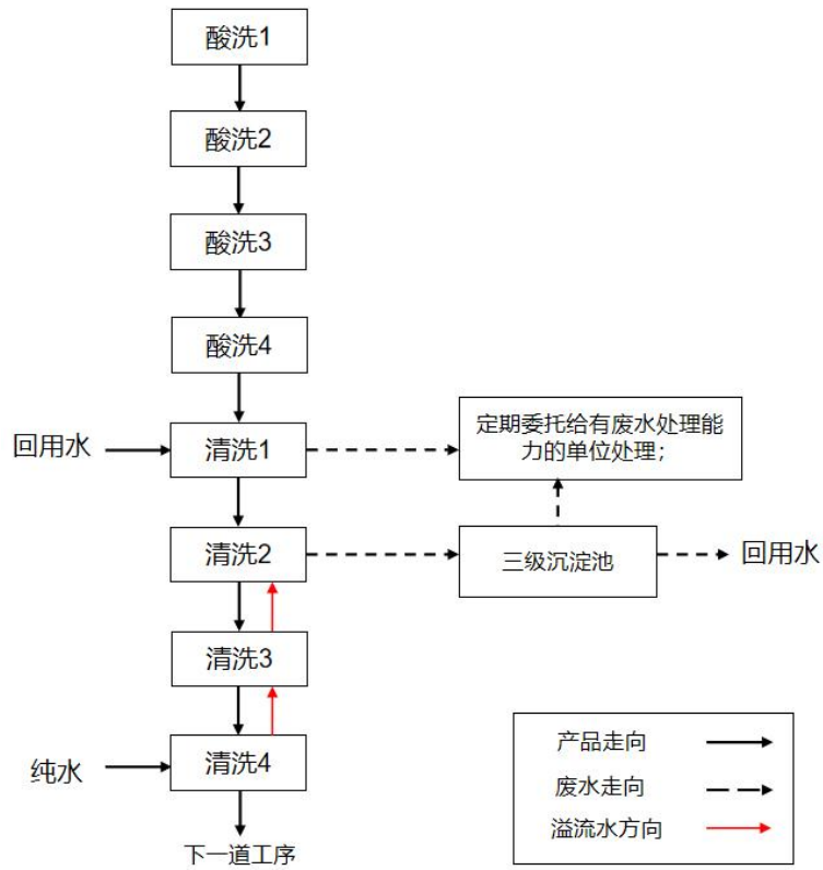
项目产品酸洗清洗线走向和清洗废水流向示意图
