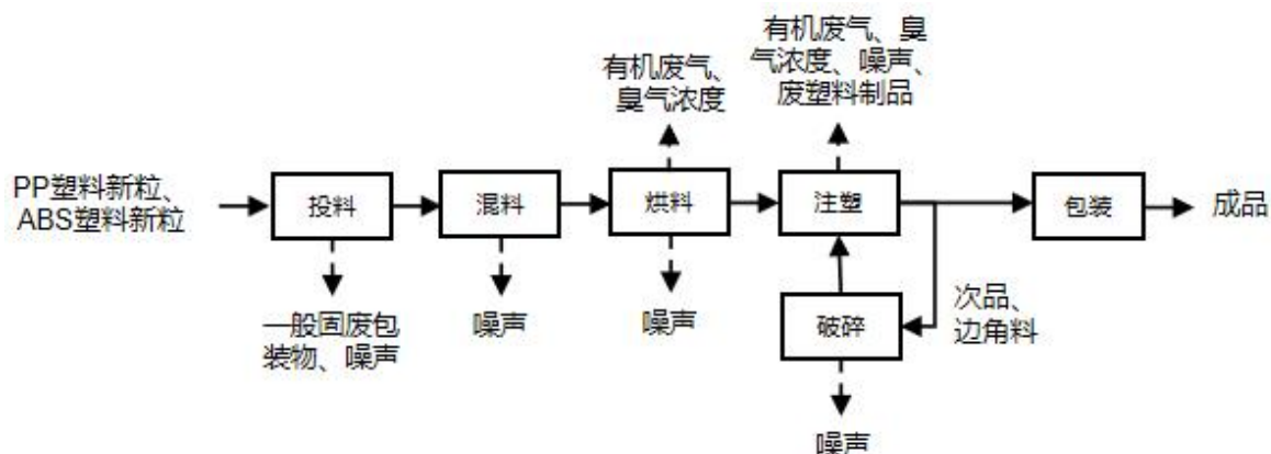
图 2-2 工艺流程图
