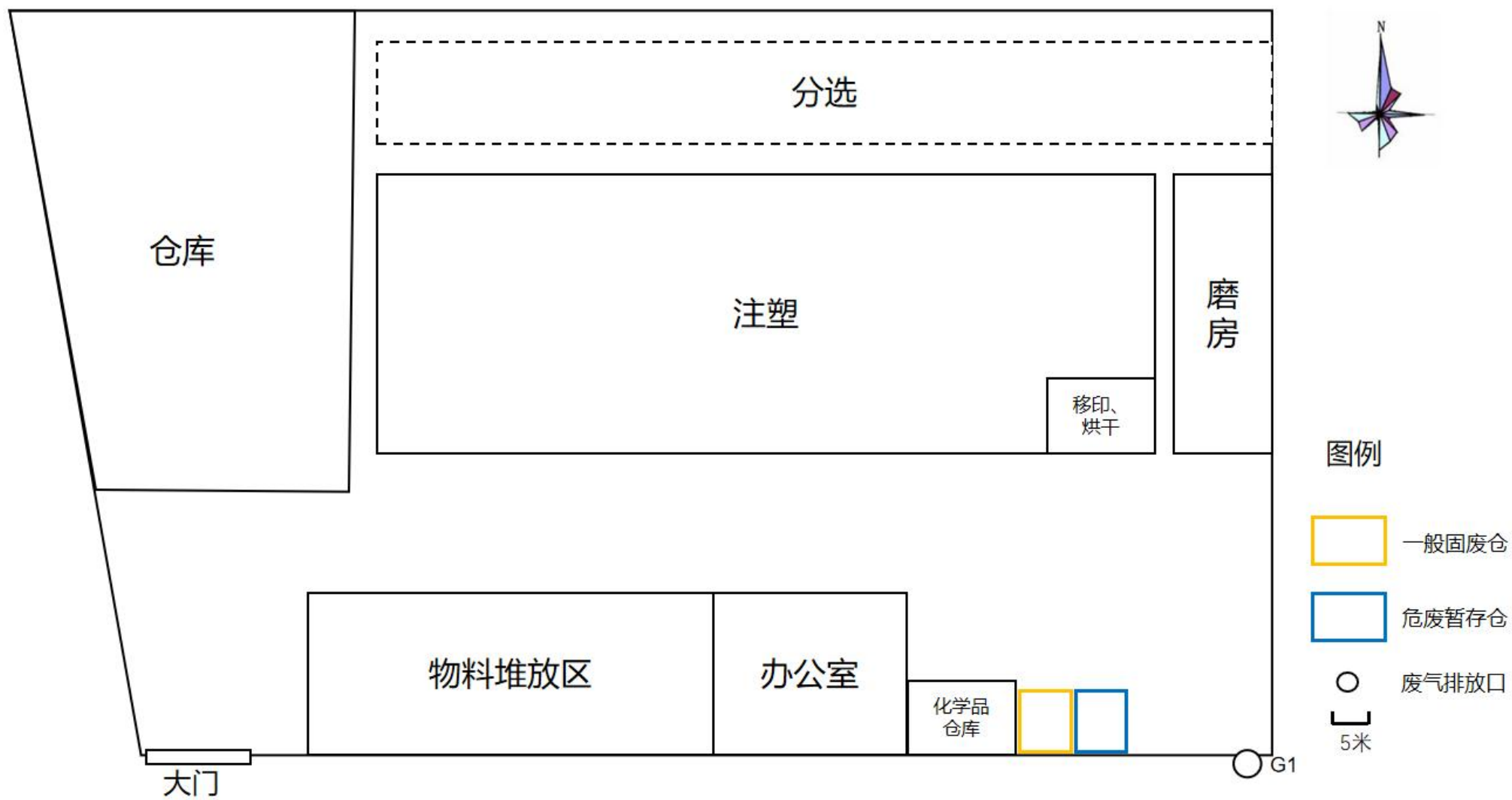
附图3 生产车间平面布置图
