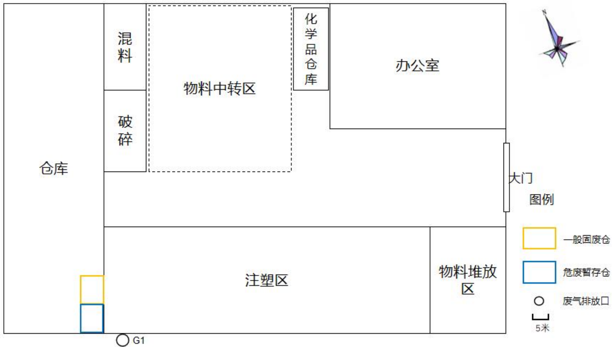
附图3 生产车间平面布置图
