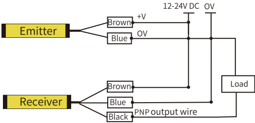
Optical-synchronization(PNP)
