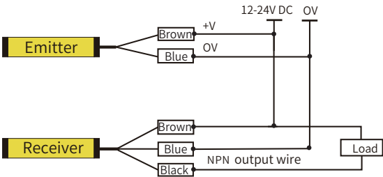
Optical-synchronization(NPN)
