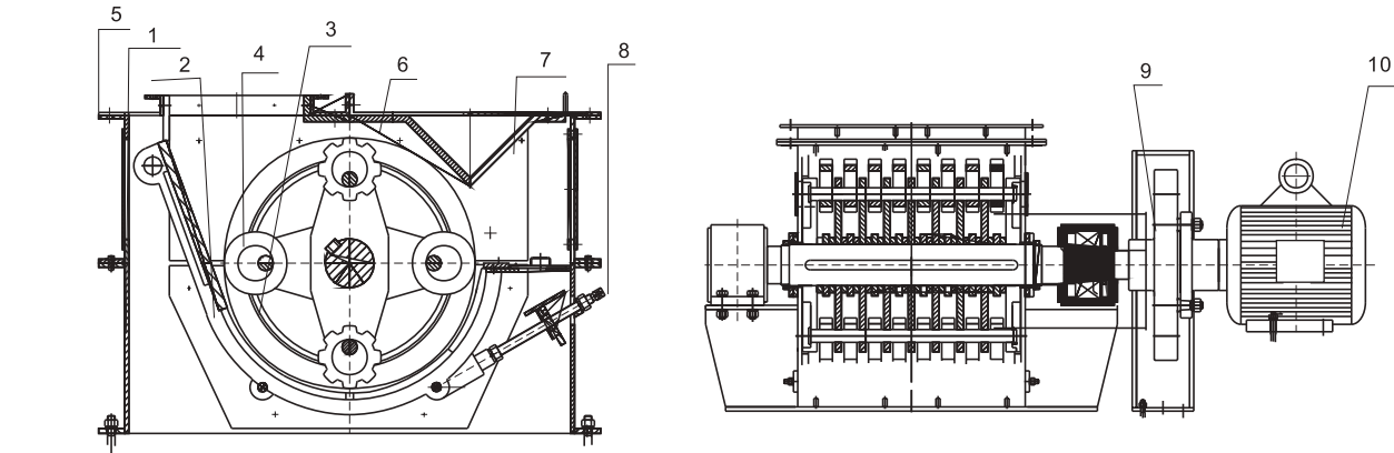
1、下机壳 2筛板机构、 3、转子 4、锤头 5、上机壳 6、上盖 7、反击板 8、调节机构 9、联轴器 10、电机
