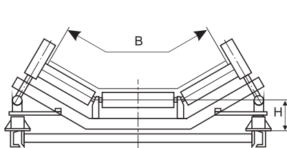
1-调心挡辊 2-拉杆 3-杠杆 4-挡辊
