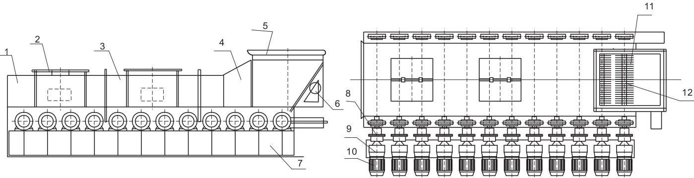
1.前机罩 2.检修罩 3.中机罩 4.连接机罩 5.进料口 6.旁路机构 7.底座 8.联轴节 9.减速机 10.电机 11.筛轴 12.筛片
