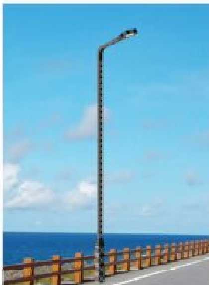
TT-4803 H=12m
