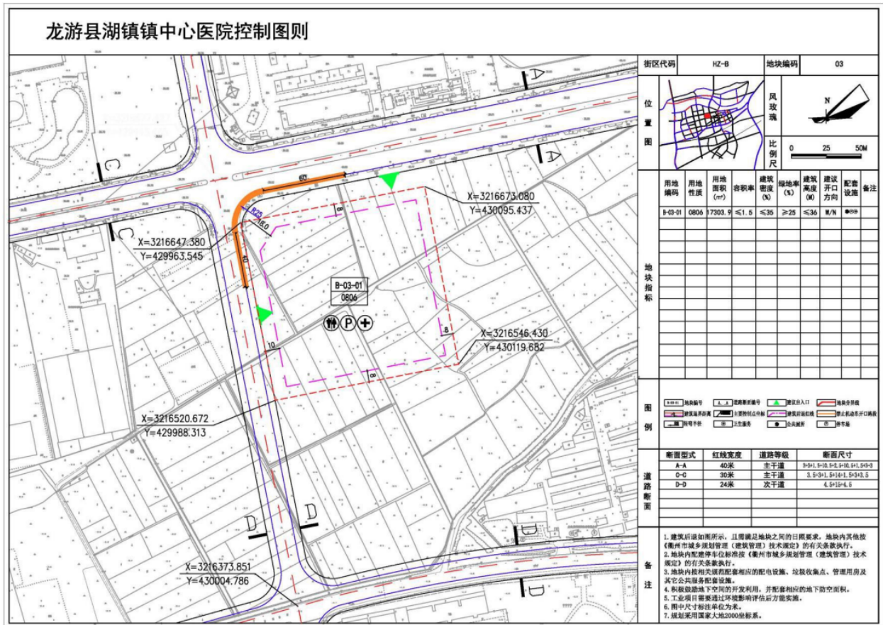
图 2.2-1 调查地块规划图
